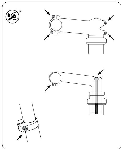
mögliche Positionen von Schraubverbindungen zur Anpassung
